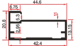
LG 111 0.430 Kg/mt
