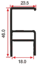
LG 356 0.633 Kg/mt
