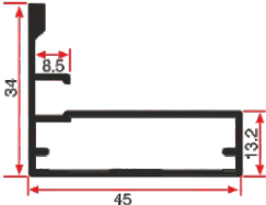
LG 112 0.480 Kg/mt
