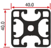
LG 801 1.830 Kg/mt
