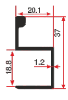
LG 361 0.295 Kg/mt
