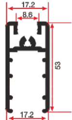
LG 433 0.355 Kg/mt Sürü Dar Alt Bağlayıcı
