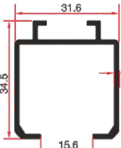
LG 325 0.470 Kg/mt
