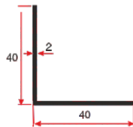
40x40 Köşebent 0.443 Kg/mt
