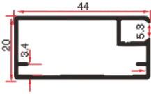
LG 109A 0.423 Kg/mt
