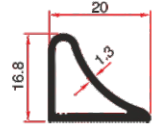
LG 371 0.214 Kg/mt
