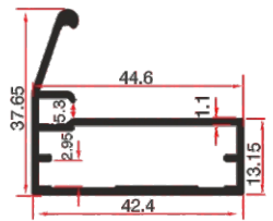
LG 115 0.525 Kg/mt
