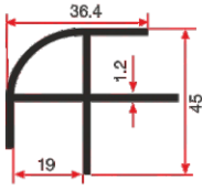
LG 251 0.486 Kg/mt
