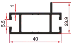
LG 821 0.380 Kg/mt
