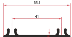
LG 440 0.267 Kg/mt
