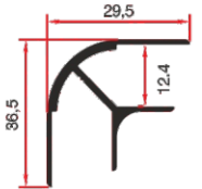
LG 254 0.315 Kg/mt
