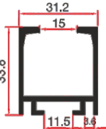
LG 326 0.567 Kg/mt
