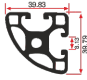
LG 808 1.489 Kg/mt
