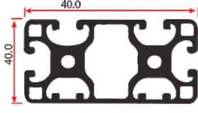
LG 803 3.125 Kg/mt
