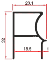
LG 362 0.281 Kg/mt
