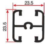
LG 403 0.328 Kg/mt
