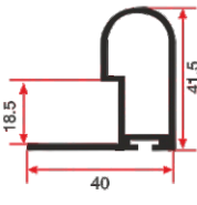
LG 351 0.591 Kg/mt
