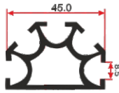
LG 817 0.900 Kg/mt
