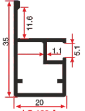
LG 103 A 0.365 Kg/mt
