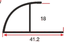
LG 256 0.315 Kg/mt
