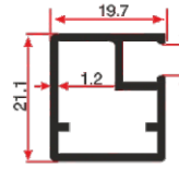
LG 103 C 0.295 Kg/mt
