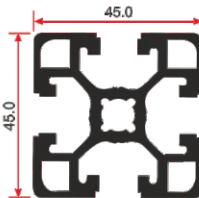
LG 807 2.059 Kg/mt
