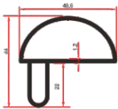
LG 180 C 0.530 Kg/mt
