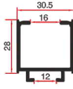
LG 327 0.445 Kg/mt
