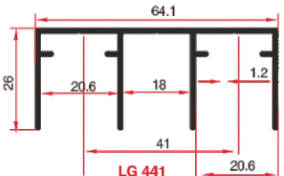
LG 441 0.573 Kg/mt
