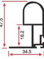
LG 357 0.707 Kg/mt
