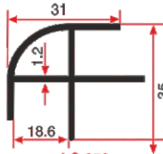
LG 252 0.330 Kg/mt
