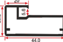
LG 110 0.450 Kg/mt
