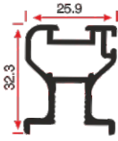
LG 400 0.458 Kg/mt
