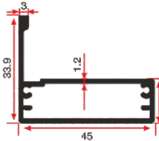
LG 114 0.485 Kg/mt
