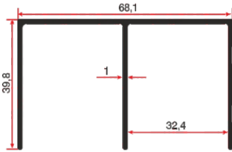
LG 409 0.535 Kg/mt
