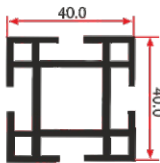
LG 805 1.080 Kg/mt
