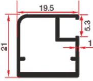
LG 100 0.290 Kg/mt
