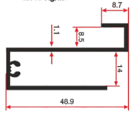
LG 416 0.280 Kg/mt
