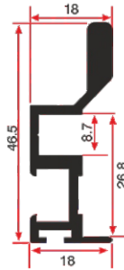
LG 419 0.630 Kg/mt
