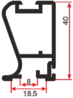
LG 430 0.450 Kg/mt Sürü Sürü Kulp Profili
