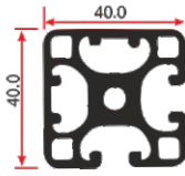
LG 802 1.835 Kg/mt
