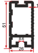
LG 401-A 0.528 Kg/mt
