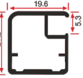
LG 101 0.291 Kg/mt
